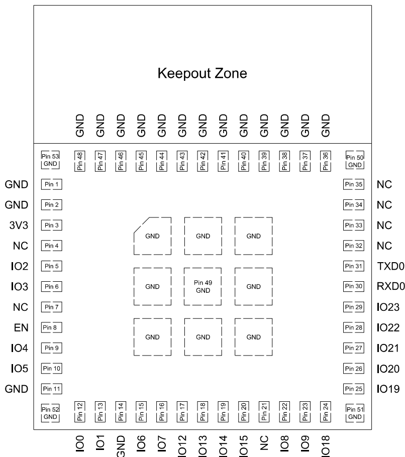
图 3-1. 管脚布局 (顶视图)
