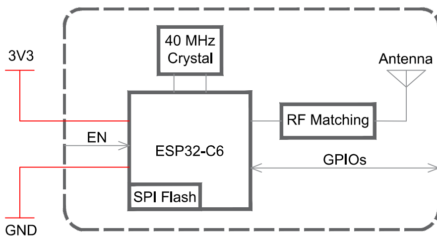
图 2-1. ESP32-C6-MINI-1 功能框图
