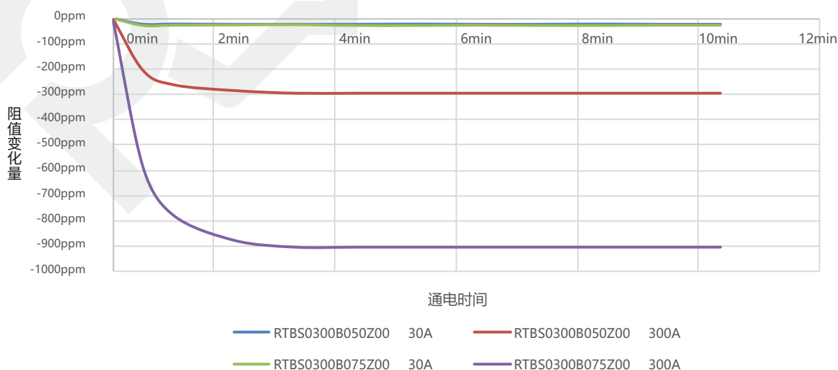
RTBS0300系列分流器通电电阻值变化情况
