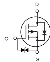
P-Channel MOSFET
