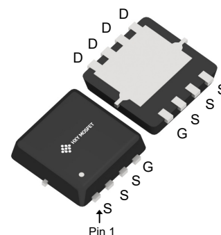
DFN3X3-8L (PowerDI3333-8)
