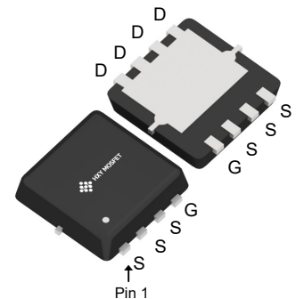
DFN3X3-8L (Power-33-8)
