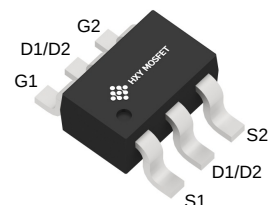
SOT-23-6L
