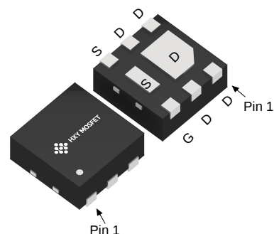
DFN2X2B-6L
