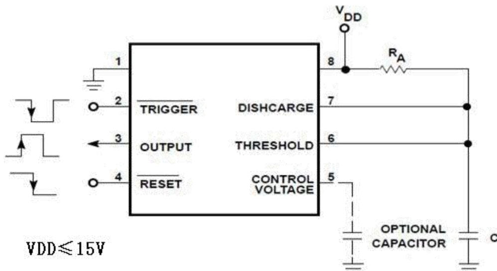
图 1：单稳态（单次）
