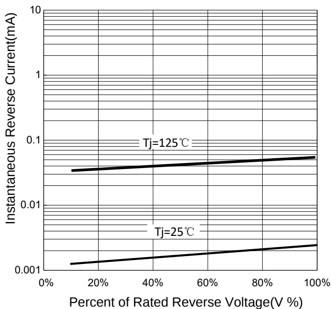
FIG 3: V_R - I_R
