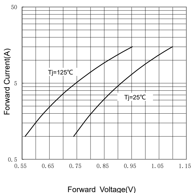
FIG 4: I_F - V_F
