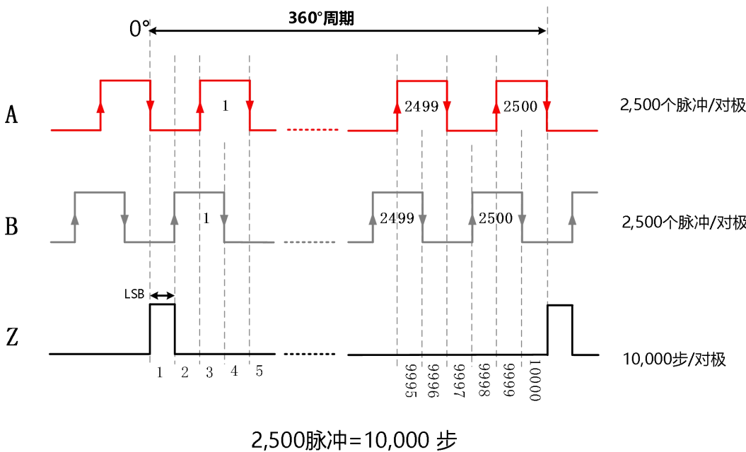
图-8: ABZ 输出分辨率=2,500 脉冲/对极
