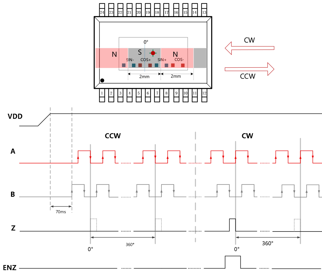
图-6: ABZ输出
