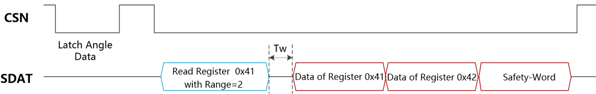
图-19: SPI 读锁存角度数据
