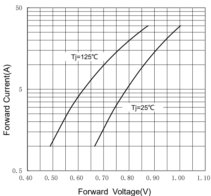
FIG 4: I_F - V_F
