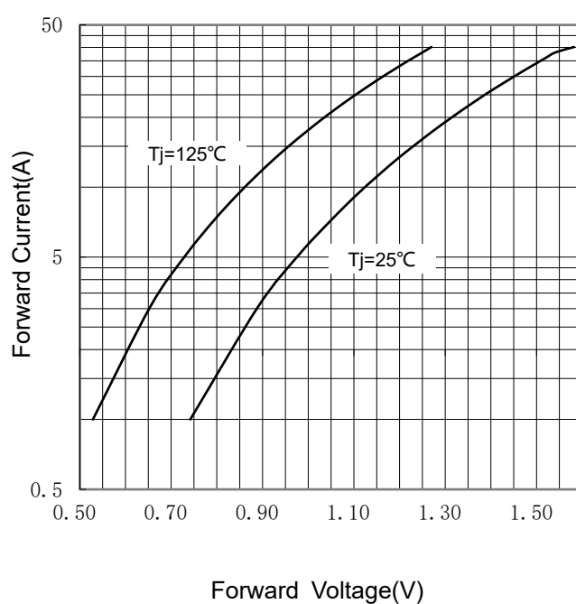
FIG 4: I_F - V_F
