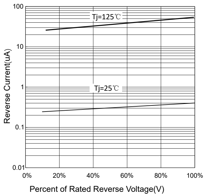
FIG 3: V_R - I_R
