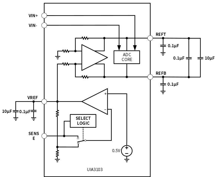
图 6-3 1.0V 内部基准电压配置
