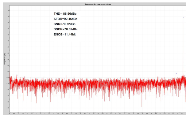
图 4-2 单音 FFT f_{IN} = 19.6MHz , f_{SAMPLE} = 40MHz
