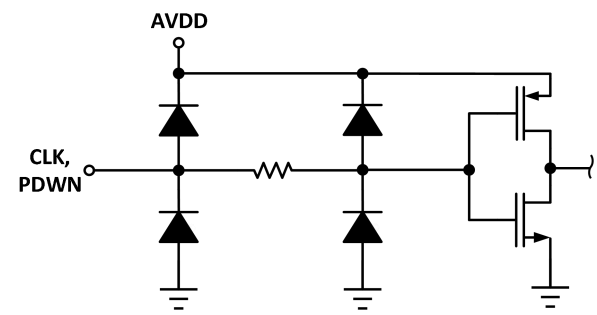
图 5-4 等效数字输入电路
