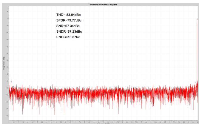
图 4-3 单音 FFT f_{IN} = 100MHz , f_{SAMPLE} = 40MHz
