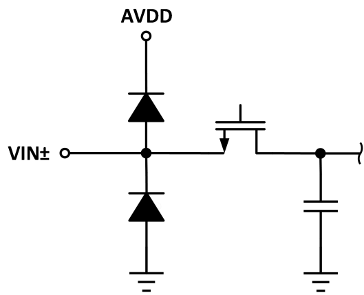
图 5-1 等效模拟输入电路
