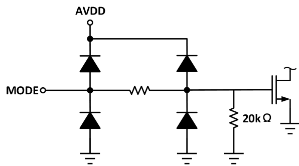
图 5-3 等效 MODE 输入电路
