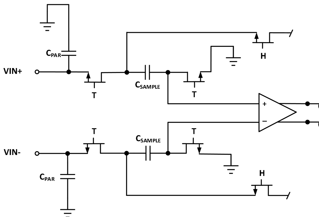
图 6-1 开关电容采样电路
