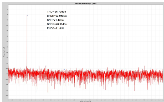
图 4-1 单音 FFT f_{IN} = 2.4MHz , f_{SAMPLE} = 40MHz
