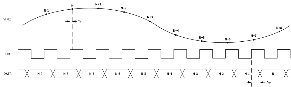
图 3-1 时序图
