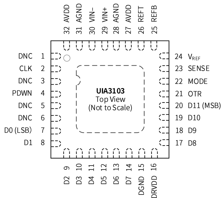
图 2-1 UIA3103 LFCSP 引脚配置
