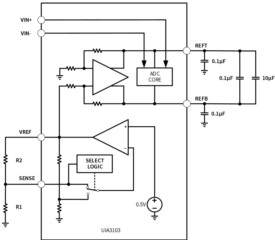
图 6-4 可编程内部基准电压配置
