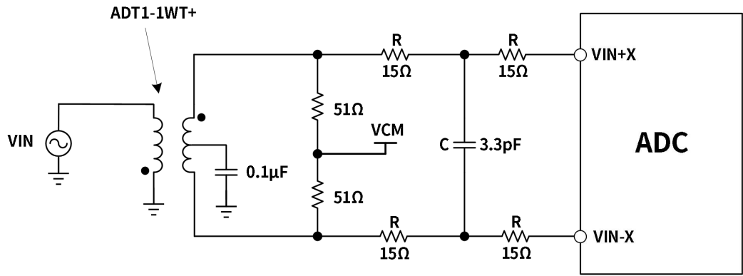
图 6-2 差分变压器耦合配置
