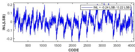
图 4-5 典型 INL
