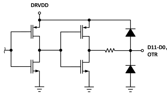
图 5-2 等效数字输出电路
