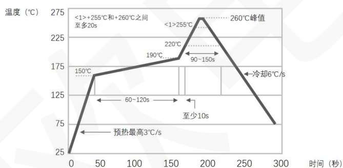
回流焊曲线图
