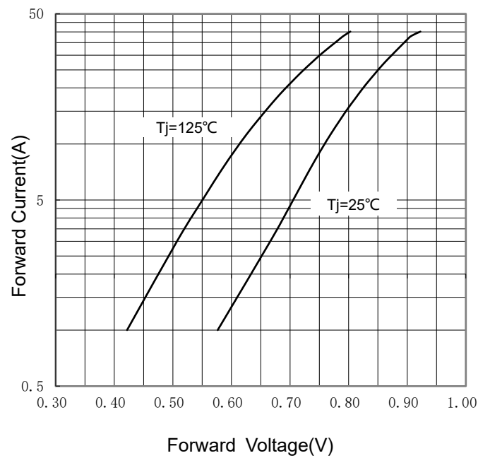
FIG 4: I_F - V_F
