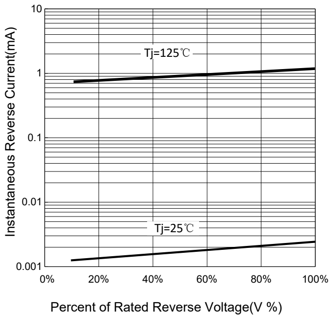
FIG 3: V_R - I_R
