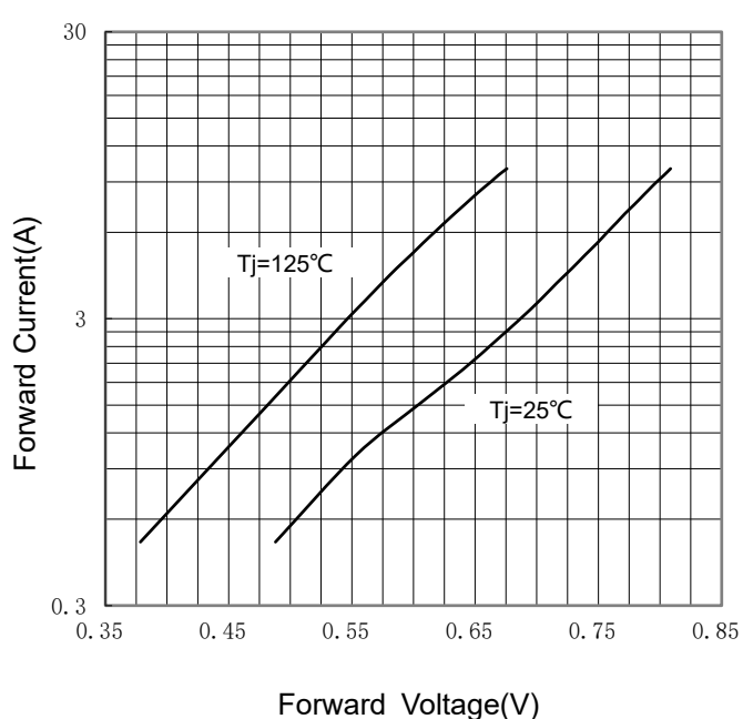
FIG 4: I_F - V_F
