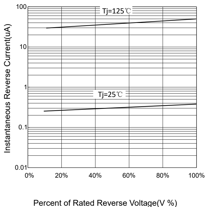
FIG 3: V_R - I_R
