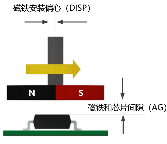
图-22: 磁铁安装
