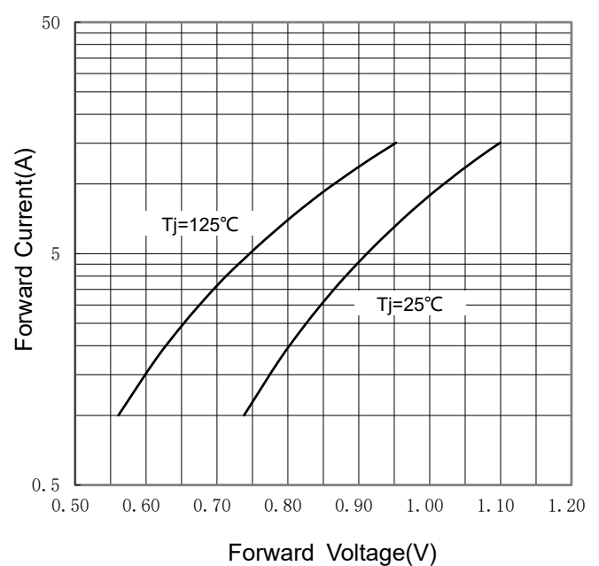
FIG 4: I_F - V_F
