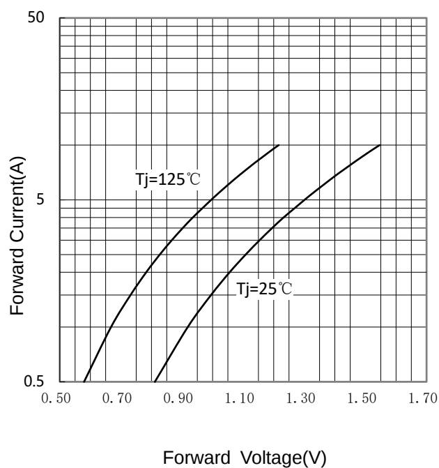
FIG 4: I_F - V_F
