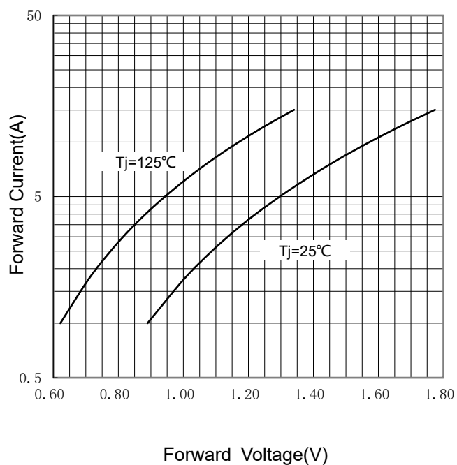
FIG 4: I_F - V_F
