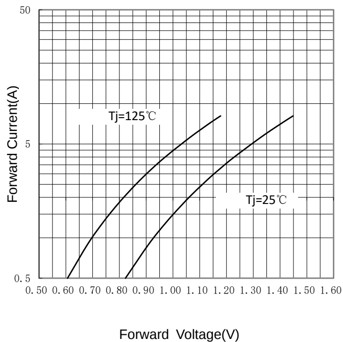
FIG 4: I_F - V_F
