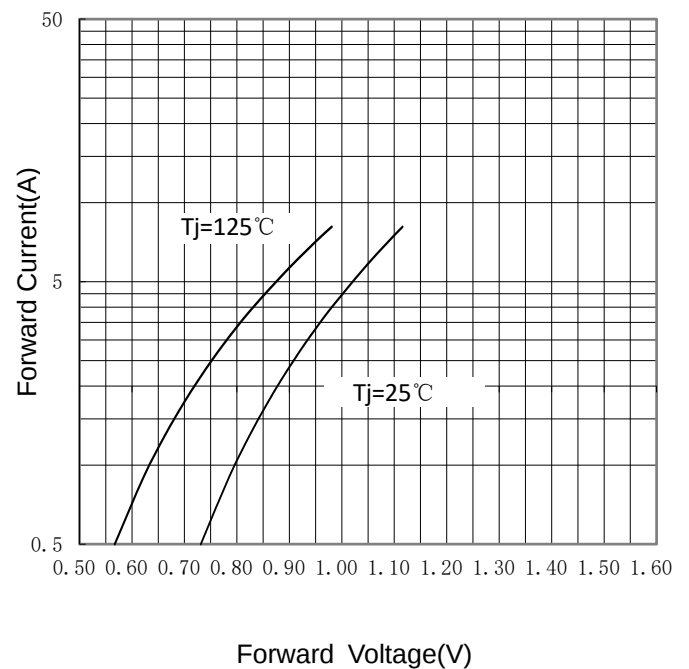
FIG 4: I_F - V_F
