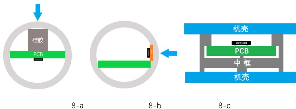
图8 ZSFS1001 按键方案示意图
