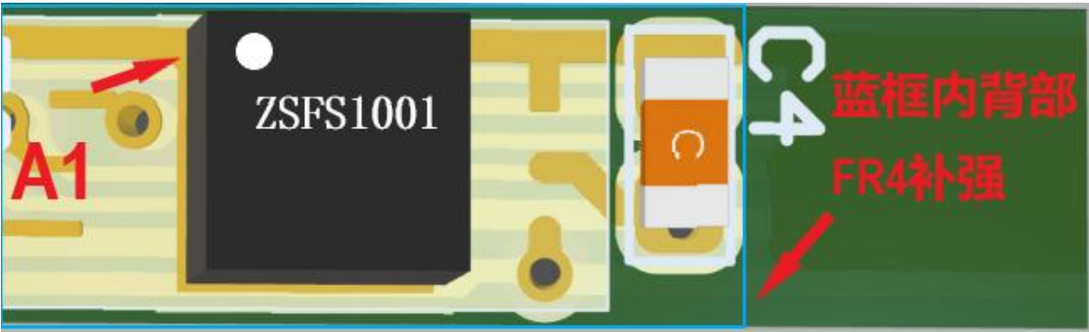
图 10 ZSFS1001 FPC 单按键结构图
