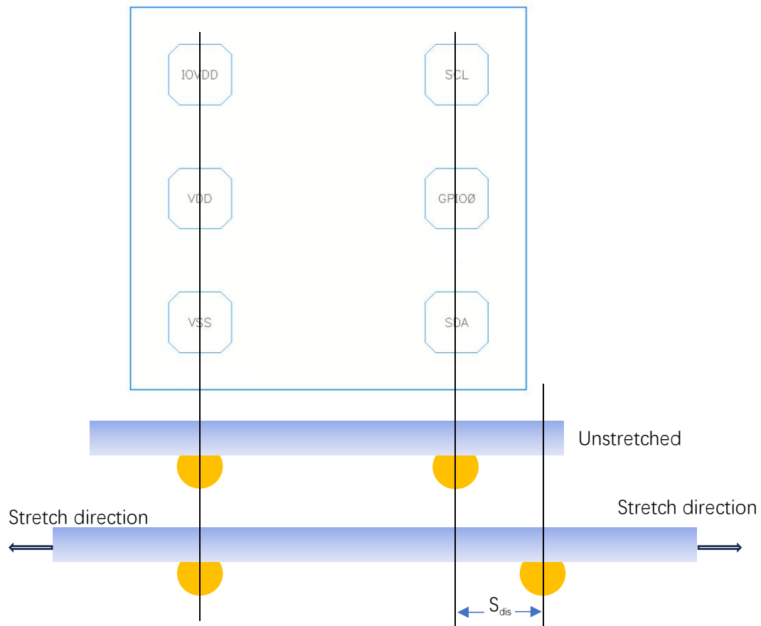
图 2 拉伸距离示意图
