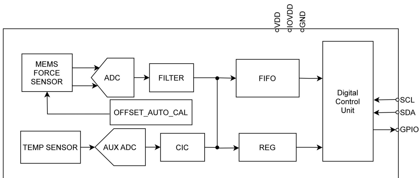
图 1. 功能框图
