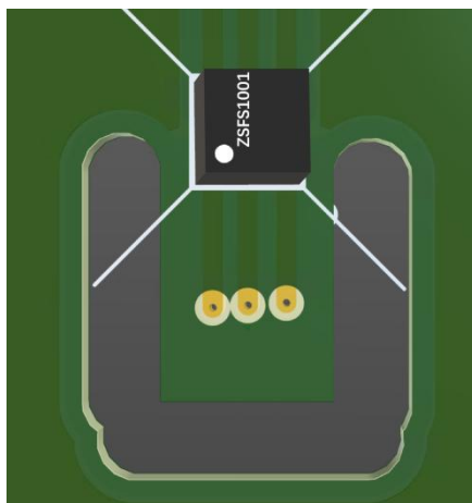
图 9-a ZSFS1001 PCB 悬臂梁结构图
