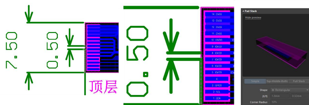
14-PIN 金手指
