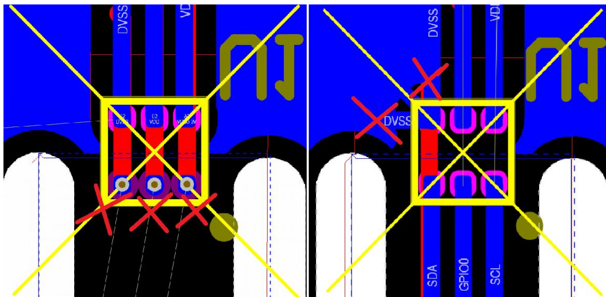
图 5-b LAYOUT 错误示意
