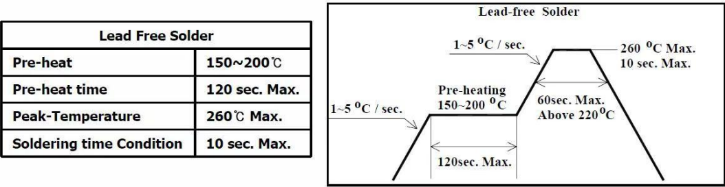
图 13 推荐回流焊曲线
