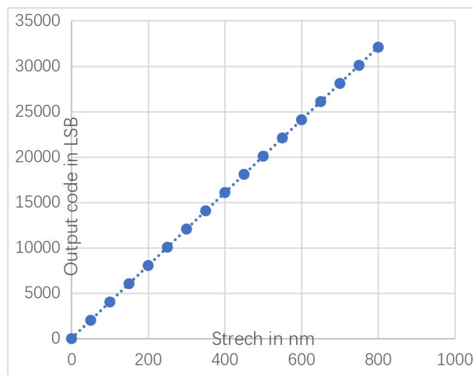
图 3 系统零点校准后拉伸距离与输出码值的对应关系图
