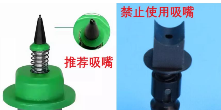
图 12 推荐使用和禁止使用吸嘴示意图
