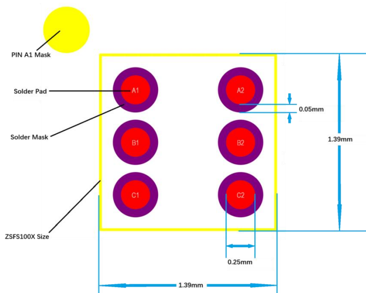
图 12 ZSFS1001 封装焊盘图
