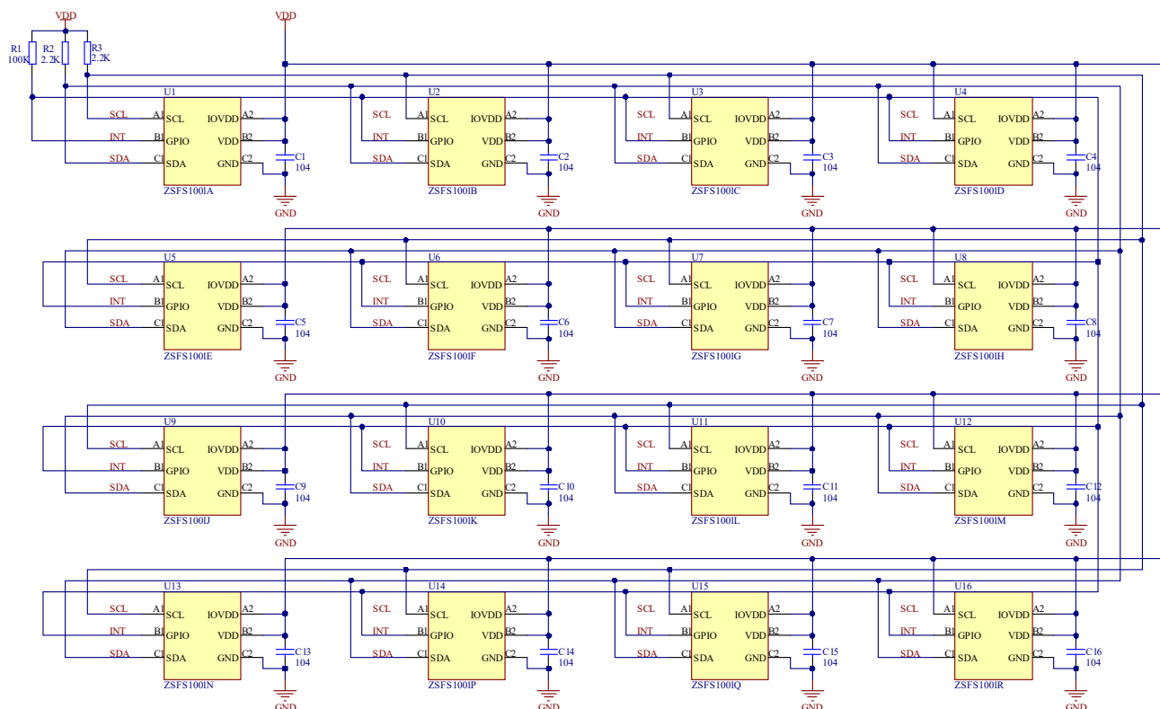
图 4-b ZSFS1001 矩阵/多按键应用参考原理图
