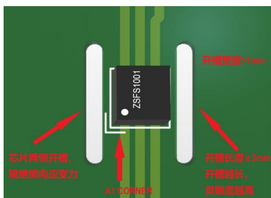
图 9-b ZSFS1001 PCB 桥式结构图
