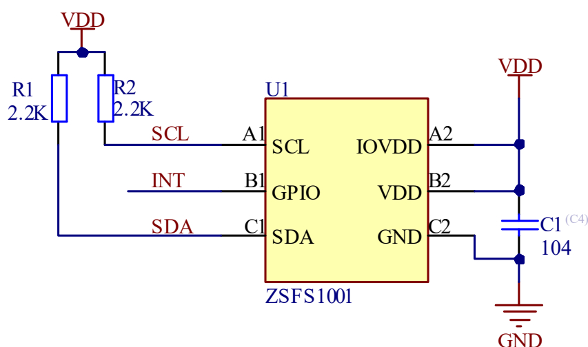
图 4-a ZSFS1001 应用参考原理图
