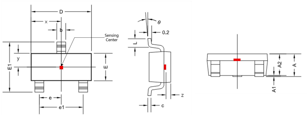
图.14 SOT-23 (Thin Outline) 封装图
