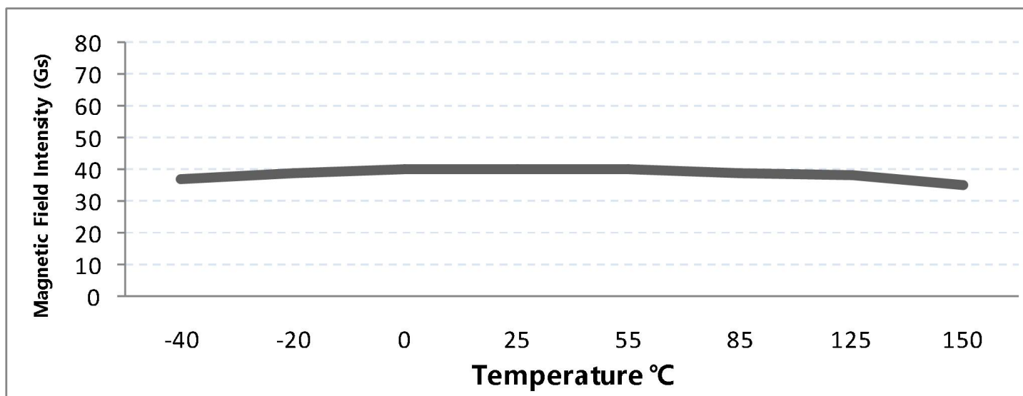
图.8 磁特性 vs. 温度 (BHYS)
