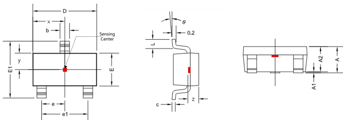
图.12 SOT-23 封装图
