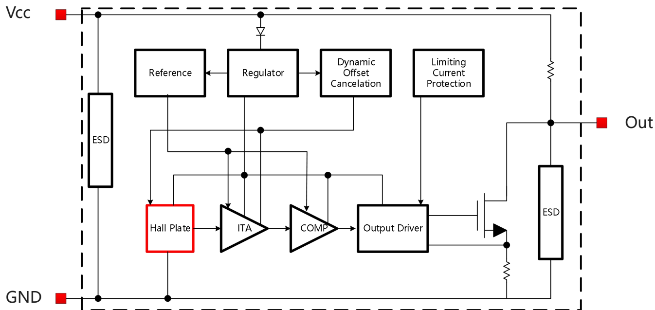
图.5 功能框图
