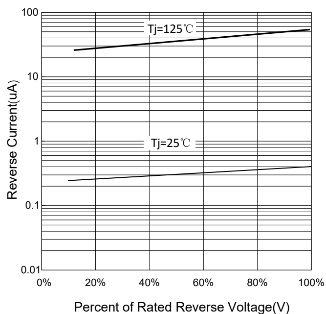
FIG 3: V_R - I_R
