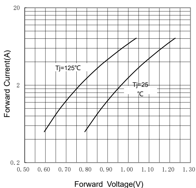
FIG 4: I_F - V_F
