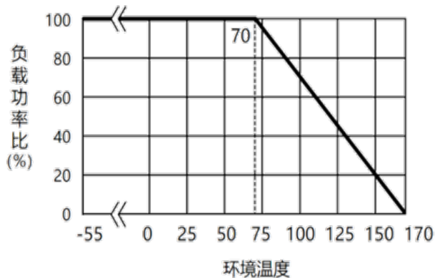
功率曲线
