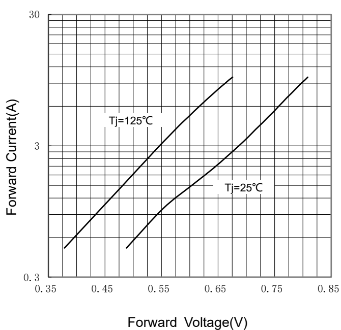
FIG 4: I_F - V_F
