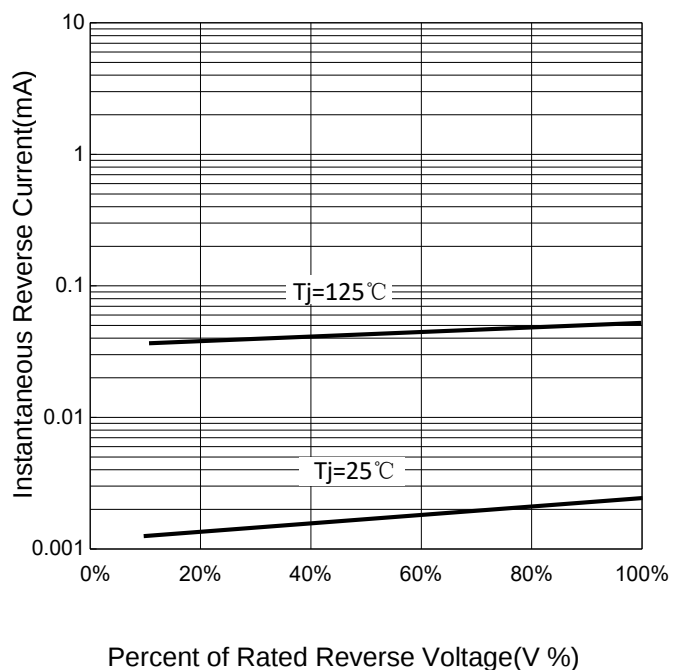
FIG 3: V_R - I_R
