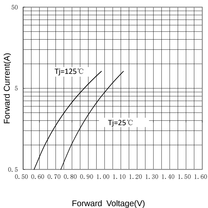
FIG 4: I_F - V_F
