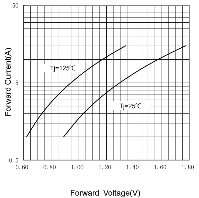
FIG 4: I_F - V_F
