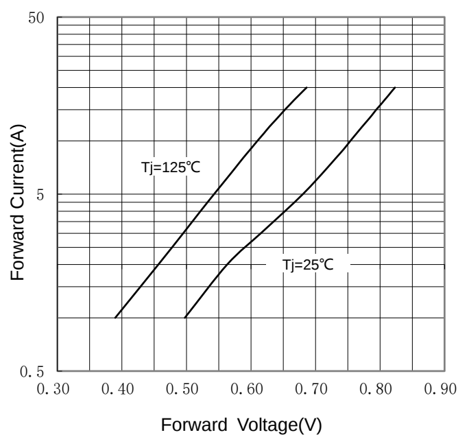
FIG 4: I_F - V_F
