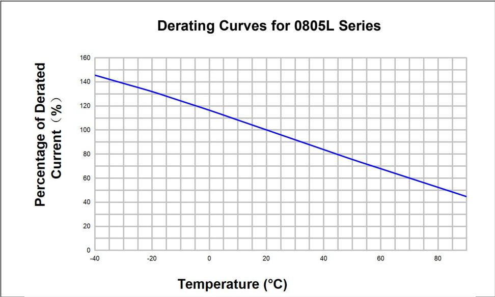
Thermal Derating Curve/环境温度与工作电流关系特性图
