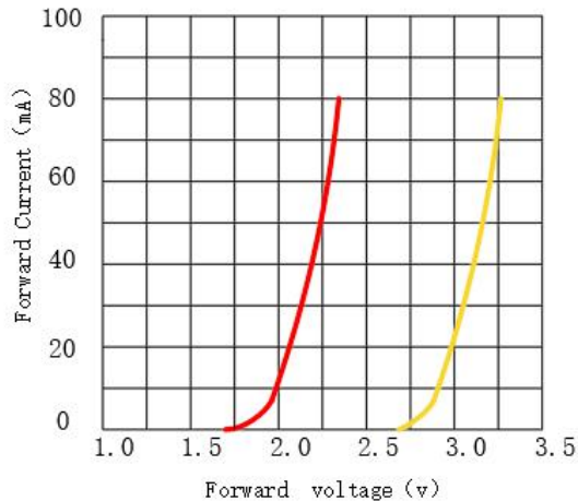
伏安特性 Volt ampere characteristic
