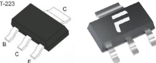
SOT-223
