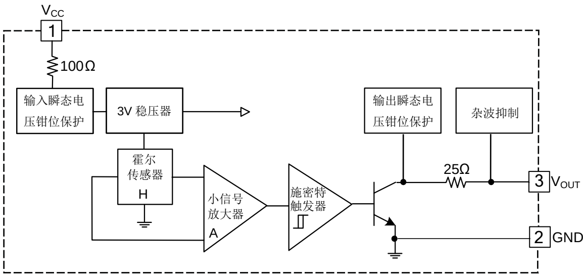
图 1, SL 3141内部结构框图
