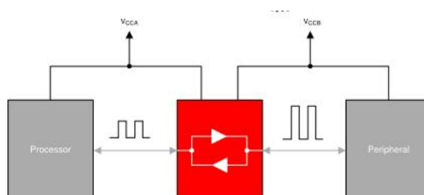
图 1 功能框图
