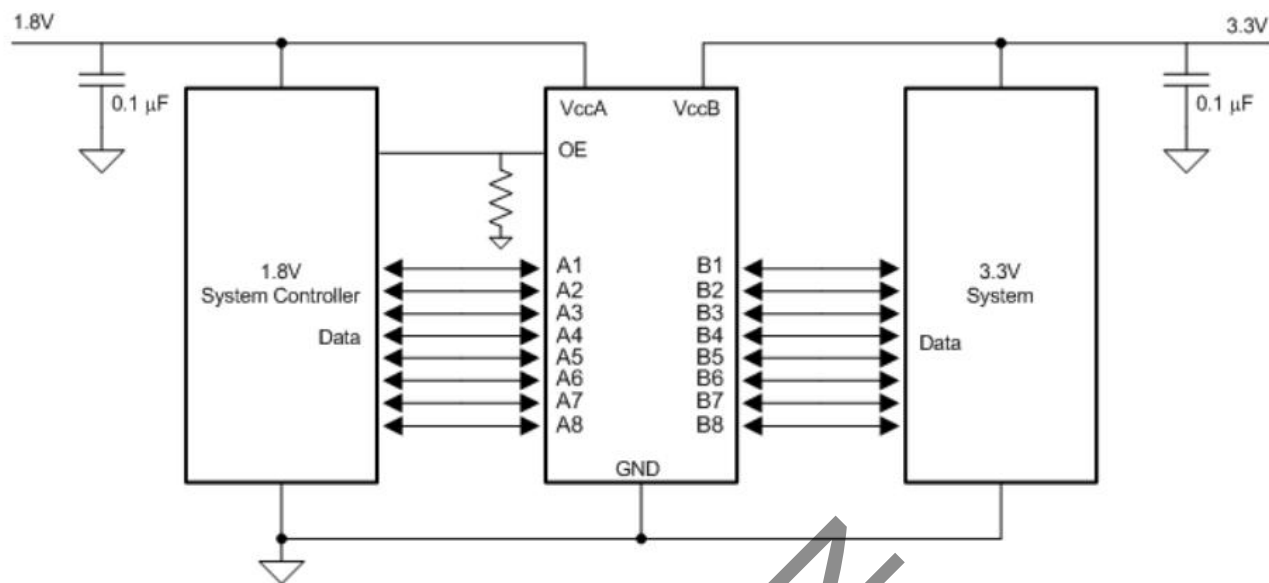
图 10 典型应用图
