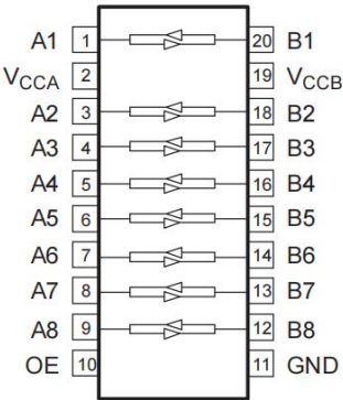
图 2 引脚排列图（顶视图）
