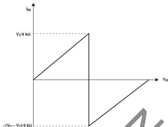
图 9 典型 I_{IN} 与 V_{IN} 曲线
