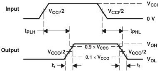
图 6 传输延迟波形图
