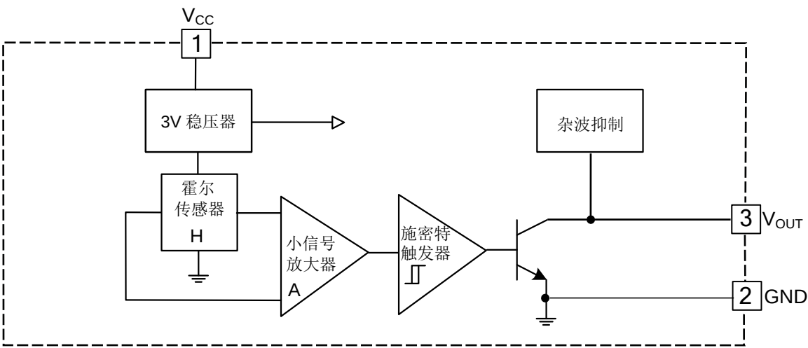
图 1, SL1713内部结构框图
