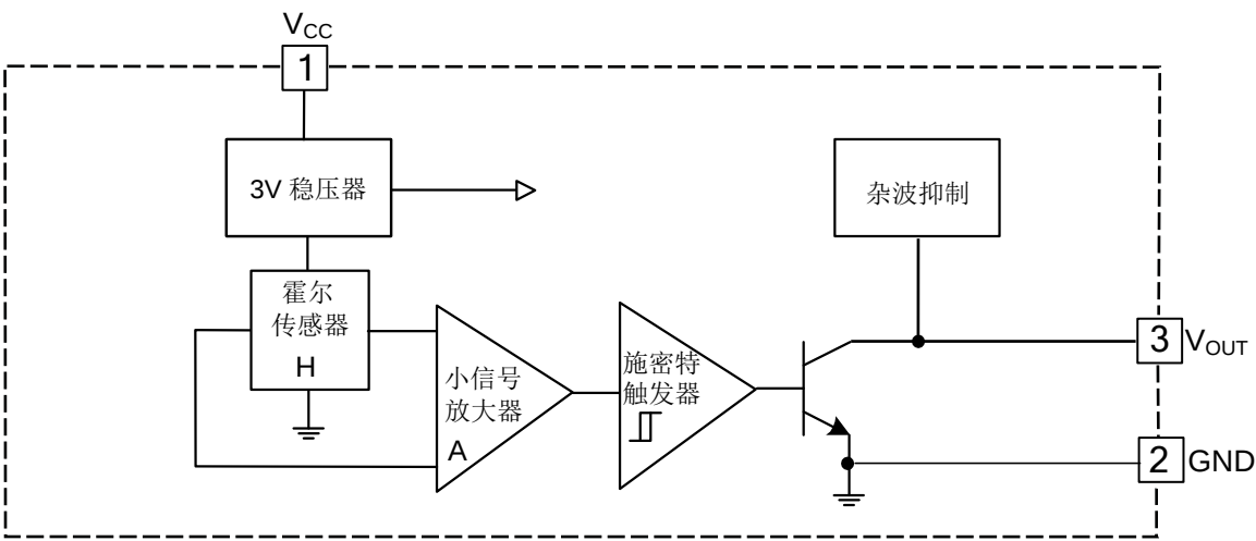
图 1, SL1715内部结构框图
