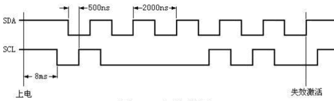
图 9. POR 失效时序图
