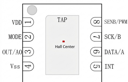
DFN-8L 封装引脚图
