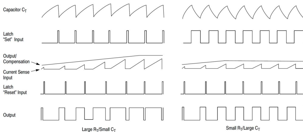
时序图
