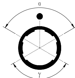
Alignment key 定位销（键位） 插头前视面视图
