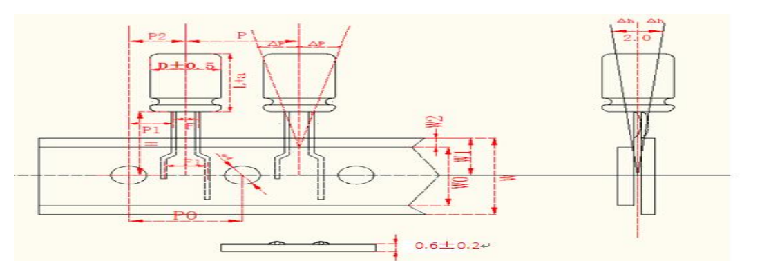
编带外型尺寸 B 图
