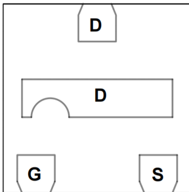
DFN1X1-3L
