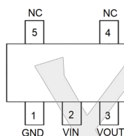
SOT23-5
