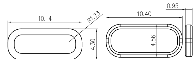
胶圈使用尺寸参考图
