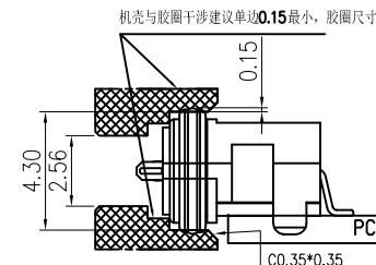
装配方向 组装示意图
