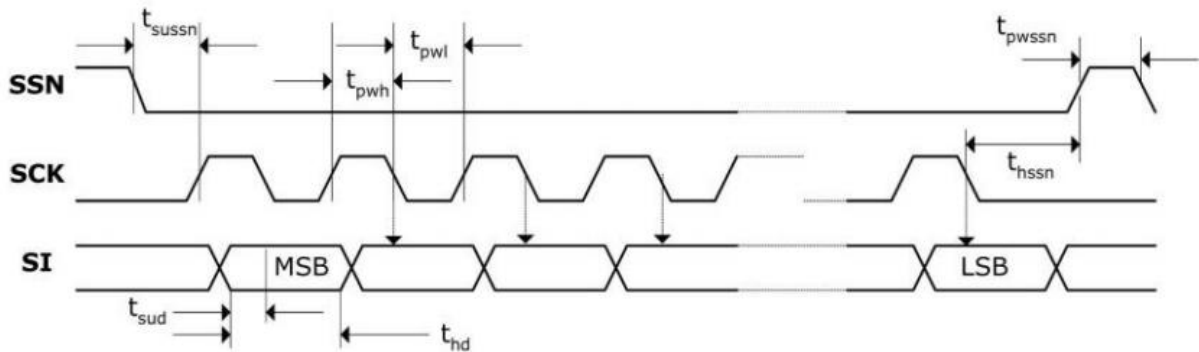
图 1. SPI 写时序
