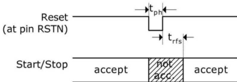
图 4. 系统复位时序
