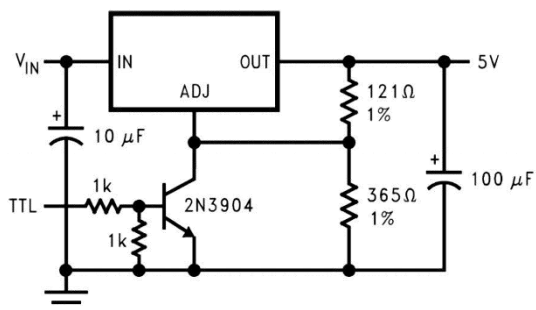
带关断的 5V 稳压器
